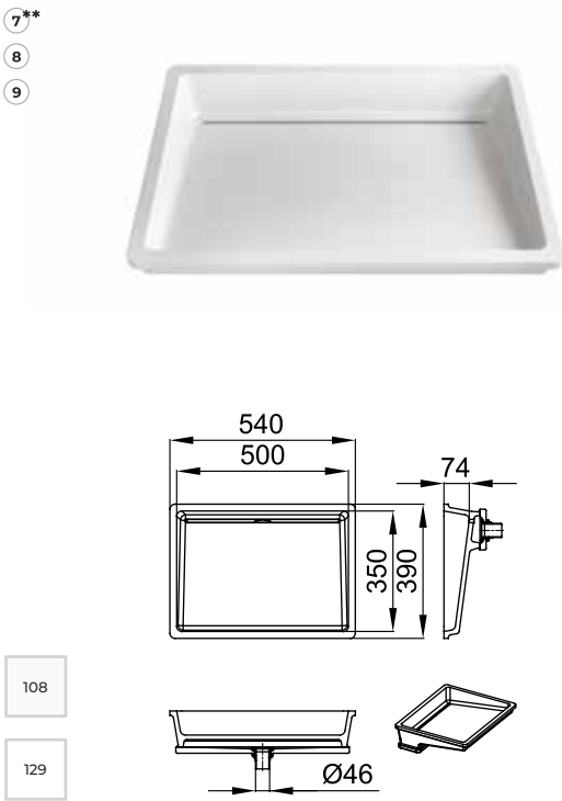
KIARA 500-UN 500 mm / 350 mm / 74 mm / ø46 mm
