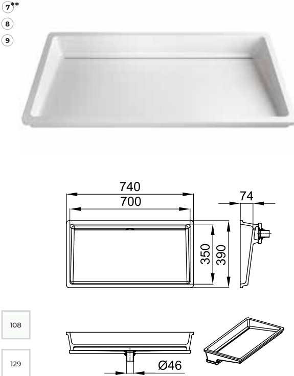
KIARA 700-UN 700 mm / 350 mm / 74 mm / ø46 mm
