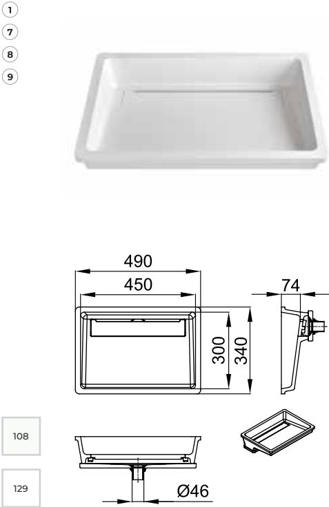
NEW KIARA 450 V-UN 450 mm / 300 mm / 74 mm / ø46 mm
